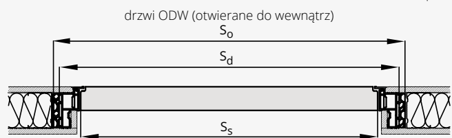
drzwi ODW (otwierane do wewnątrz)
